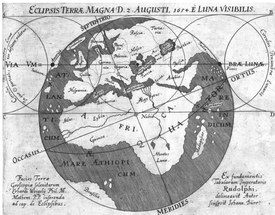
Zeichnung (Kupferstich) mit dem weltweiten Verlauf der Sonnenfinsternis am 2./12.8.1654 (aus Erhard Weigel: Secundae Partis Geoscopiae Selenitarum Disputatio Secunda De Eclipsibus [...], Jena 1654)
